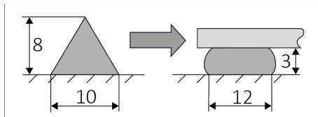
Obrázok 1: Stlačenie pásu lepidla do konečnej veľkosti
