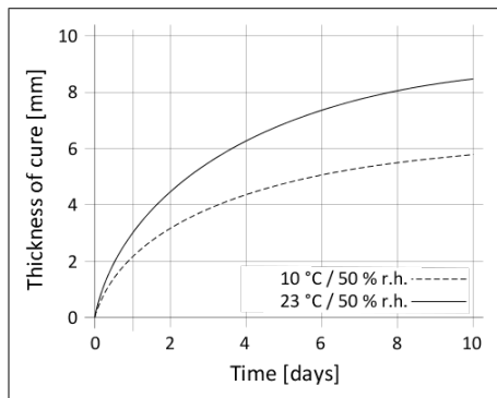
Graf 1: Rýchlosť vytvrdzovania Sikaflex®-545
